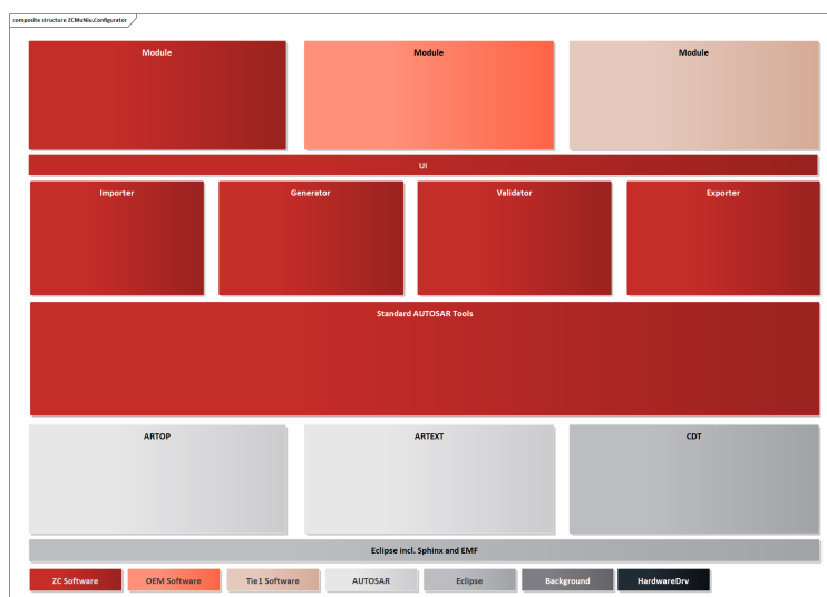
木牛配置工具架构图
